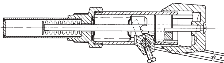
Регулятор "THERMOMAT RT-C"
